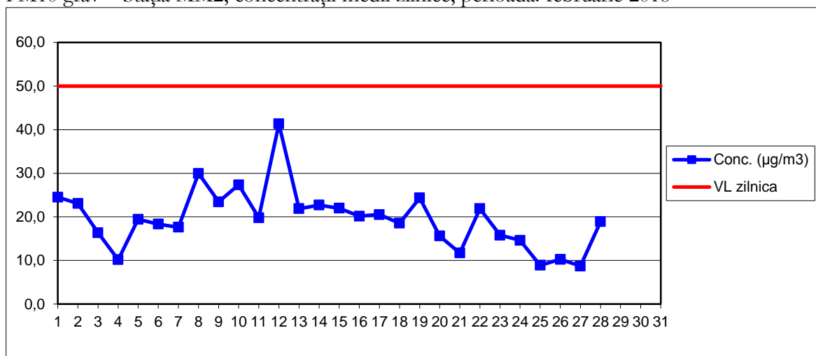
PM10 grav – Stația MM2, concentrații medii zilnice, perioada: februarie 2018
