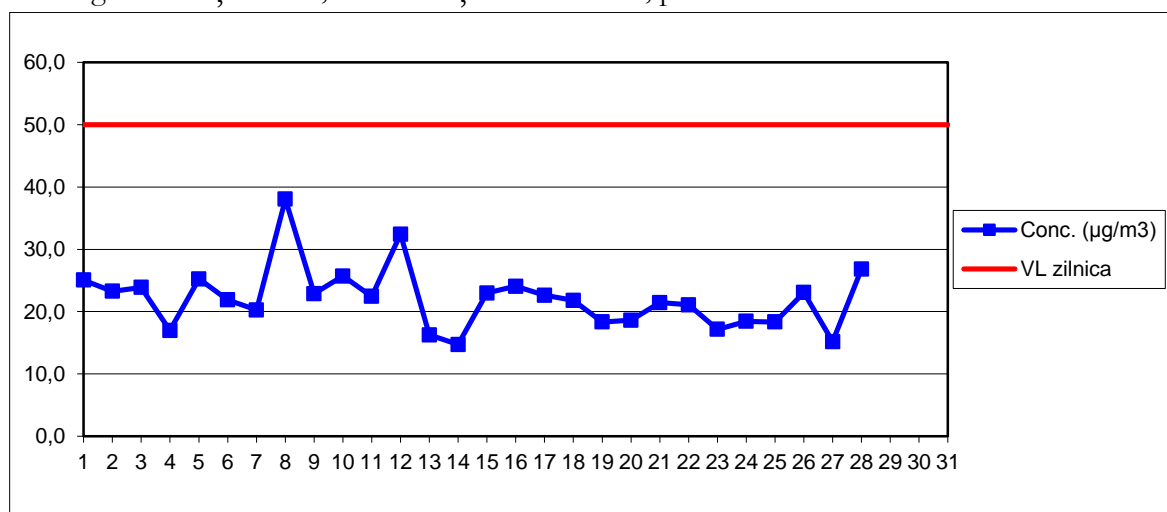
PM10 grav – Stația MM5, concentrații medii zilnice, perioada: februarie 2018
