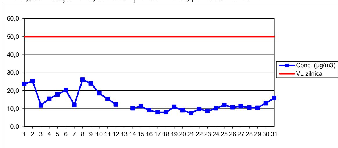
PM10 grav – Stația MM5, concentrații medii zilnice, perioada: mai 2018
