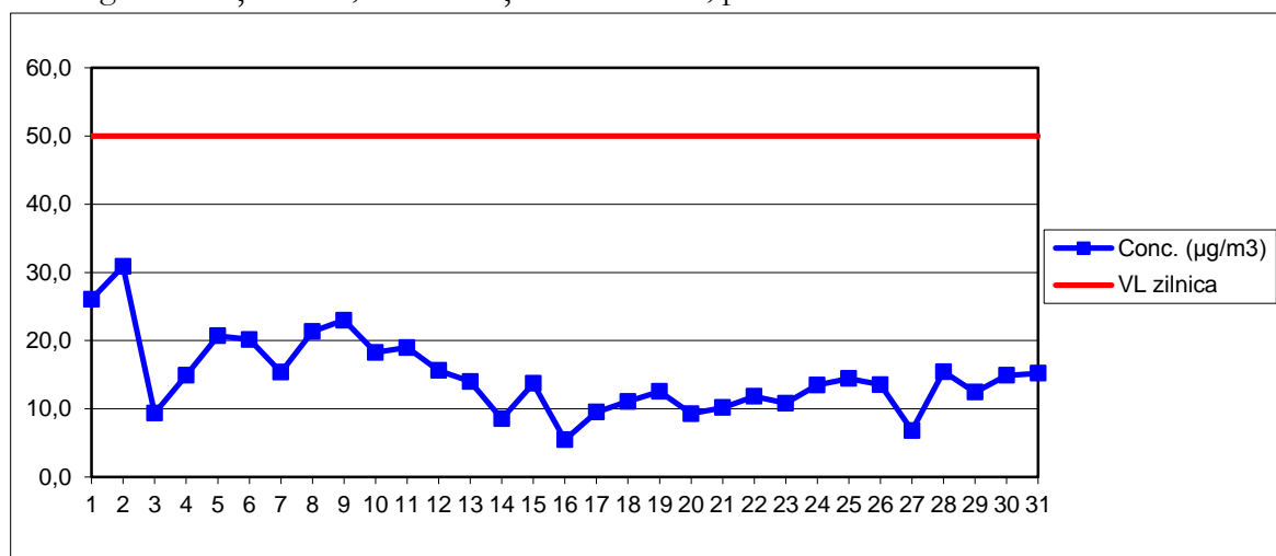
PM10 grav – Stația MM5, concentrații medii zilnice, perioada: mai 2018
