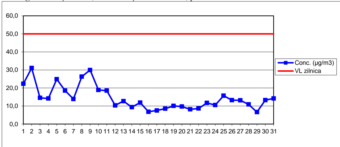
PM10 grav – Stația MM2, concentrații medii zilnice, perioada: mai 2018
