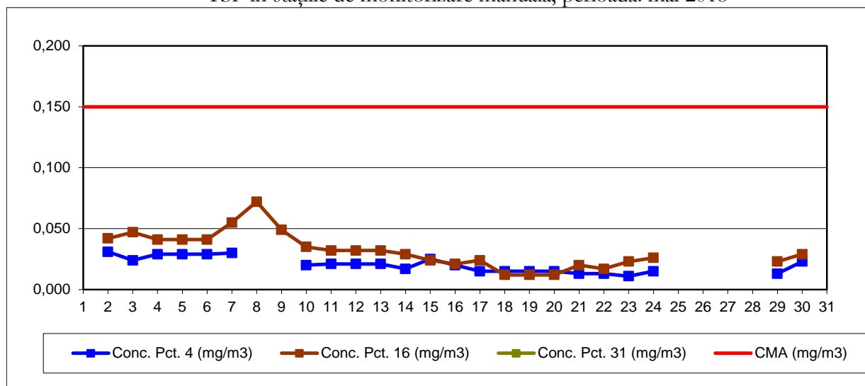
TSP in stațiile de monitorizare manuală, perioada: mai 2018
