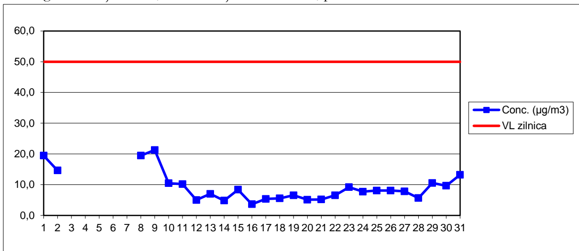
PM10 grav – Stația MM3, concentrații medii zilnice, perioada: mai 2018
