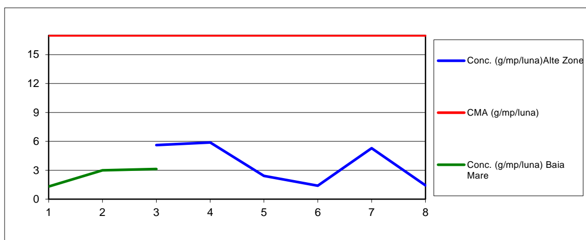
Pulberi sedimentabile - mai 2018
