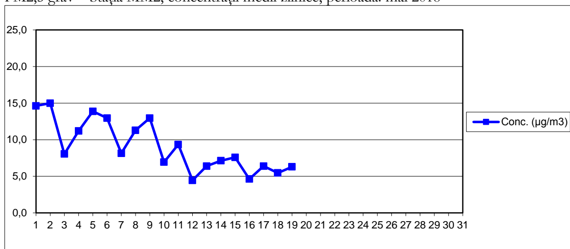
PM2,5 grav – Stația MM2, concentrații medii zilnice, perioada: mai 2018
