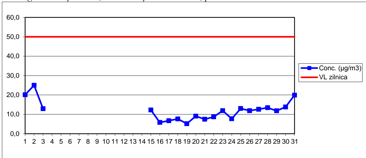
PM10 grav – Stația MM1, concentrații medii zilnice, perioada: mai 2018
