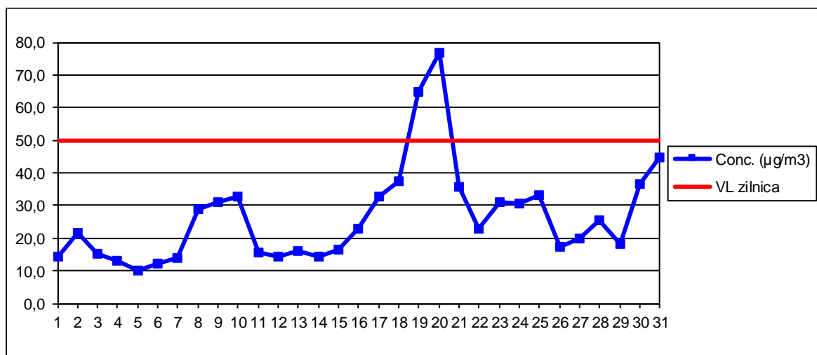
PM10 grav – Stația MM3, concentrații medii zilnice, perioada: octombrie 2018
