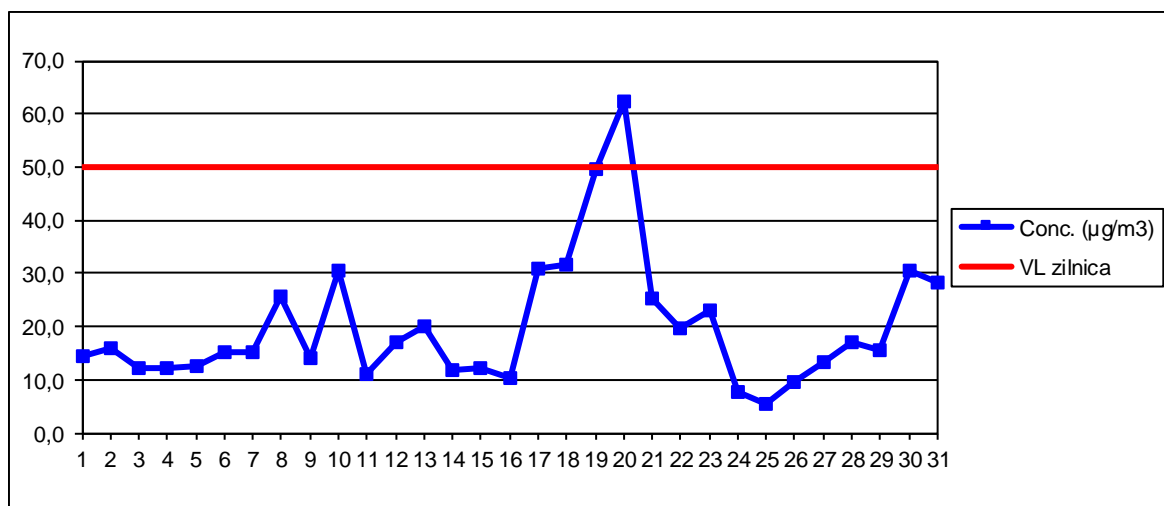
PM10 grav – Stația MM2, concentrații medii zilnice, perioada: octombrie 2018
