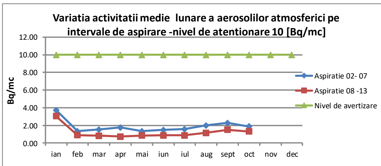
Fig. 1.3.1. Activitatea beta globală pentru aerosoli atmosferici
