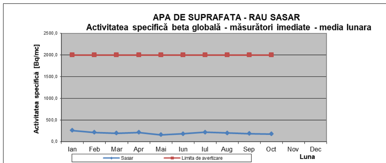
Fig. 1.4.5. Activitatea beta globală imediată pentru apa de suprafață din Râul Săsar (Pod Catedrala)
