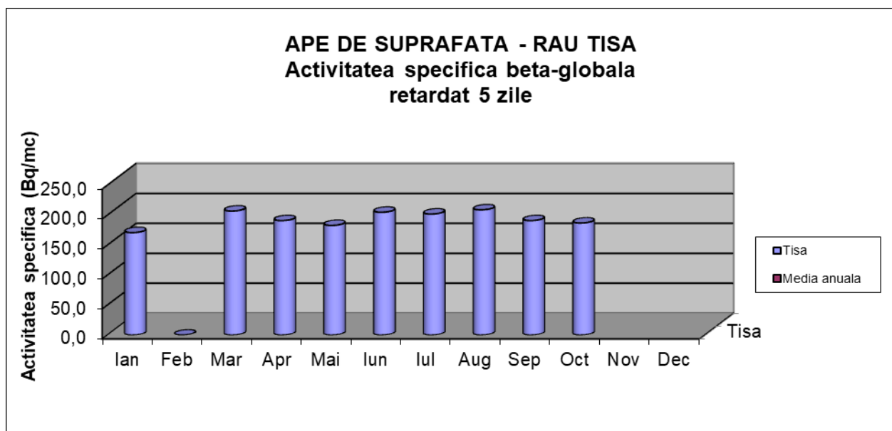
Fig. 1.3.7. Activitatea beta globală măsurată retard la 5 zile pentru apa de suprafață - Râul Tisa
