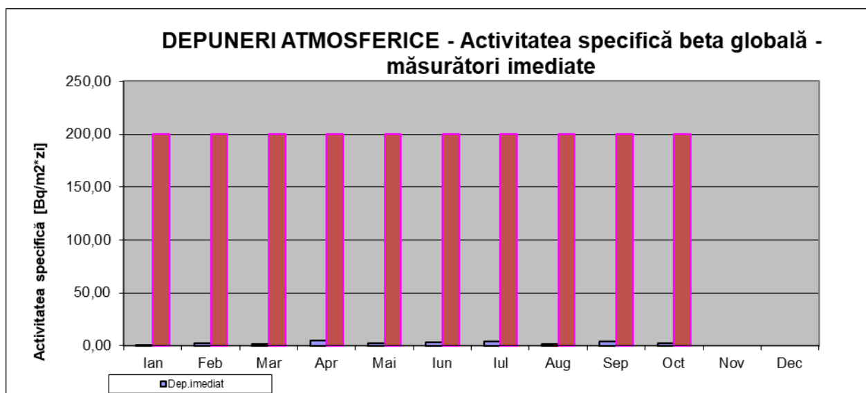
Fig. 1.3.4. Activitatea beta globală pentru depuneri atmosferice
