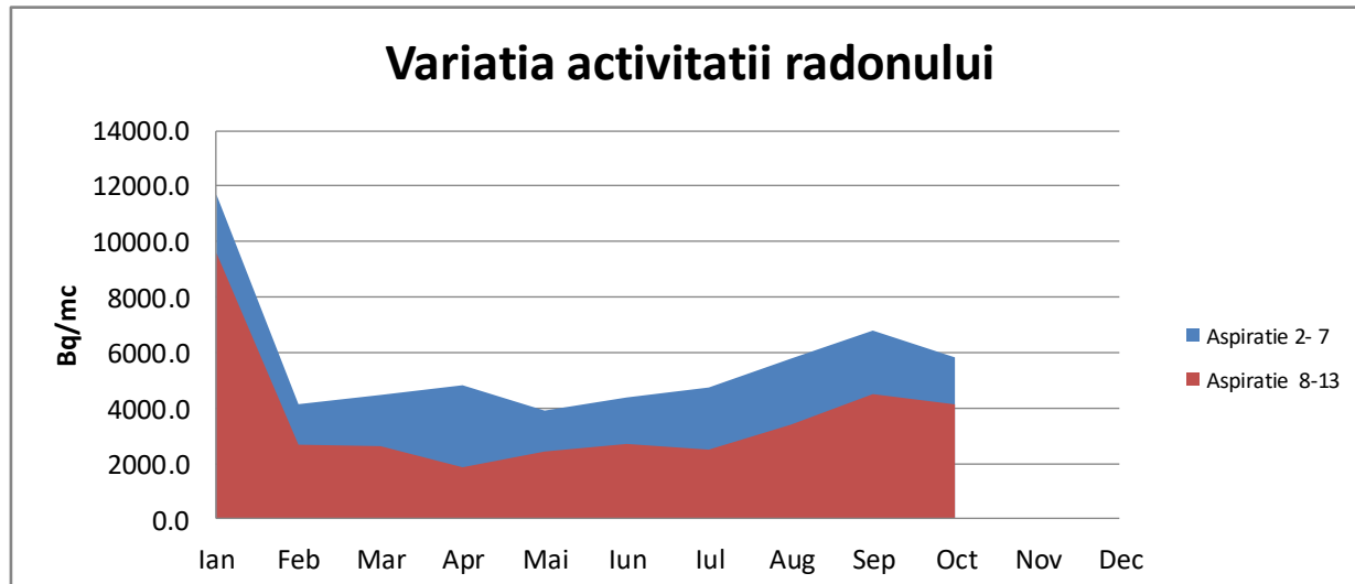
Fig. 1.3.2. Activitatea calculată a Radonului
