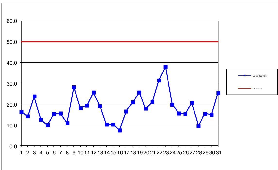
Evoluția indicatorului PM10 grav – Stația MM4, concentrații medii zilnice
