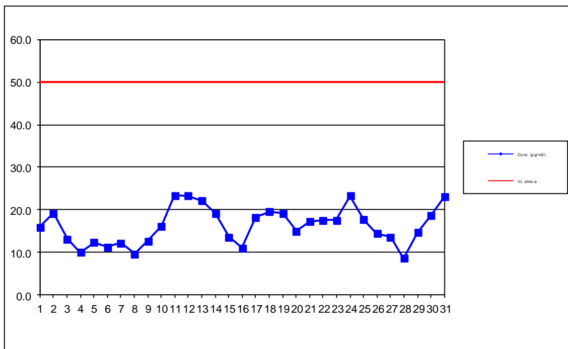
Evoluția indicatorului PM10 grav – Stația MM5, concentrații medii zilnice
