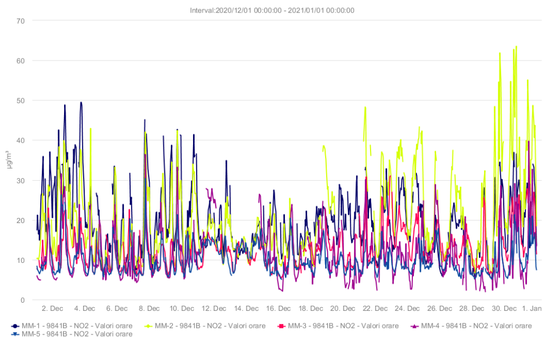
Evoluția indicatorului NO 2 – medii orare
