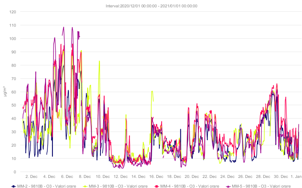
Evoluția indicatorului O 3 – medii orare
