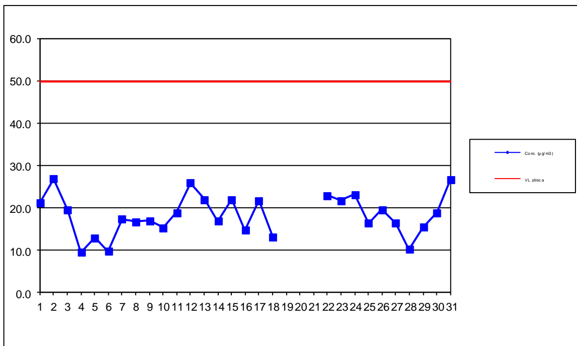
Evoluția indicatorului PM10 grav – Stația MM3, concentrații medii zilnice
