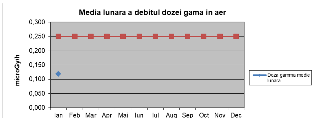
Fig. 1.3.2. Debitul dozei gamma în aer
