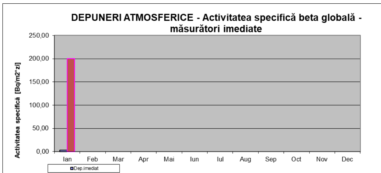
Fig. 1.3.3. Activitatea beta globală pentru depuneri atmosferice
