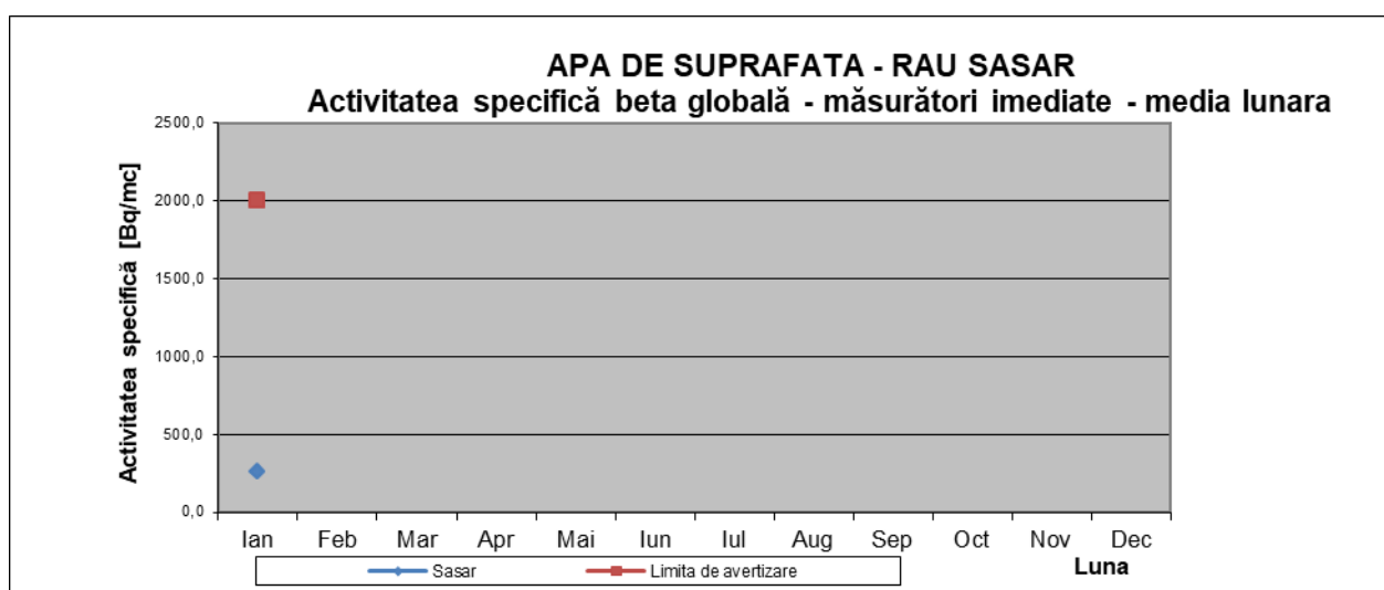
Fig. 1.3.4. Activitatea beta globală imediată pentru apa de suprafață din Râul Săsar (Pod Catedrala)
