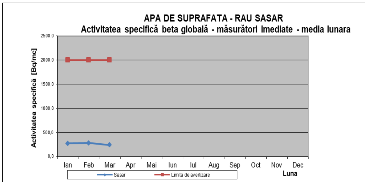
Fig. 2.4.5. Activitatea beta globală imediată pentru apa de suprafață din Râul Săsar (Pod Catedrala)
