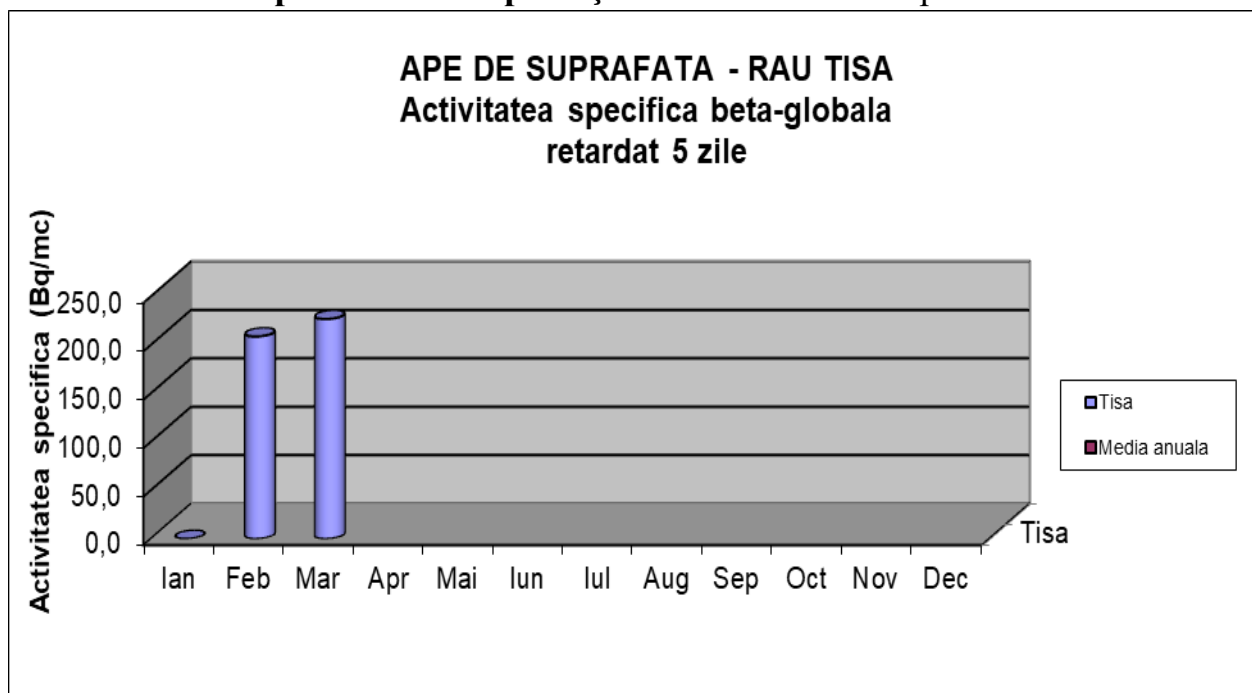
Fig. 2.3.7. Activitatea beta globală măsurată retard la 5 zile pentru apa de suprafață - Râul Tisa
