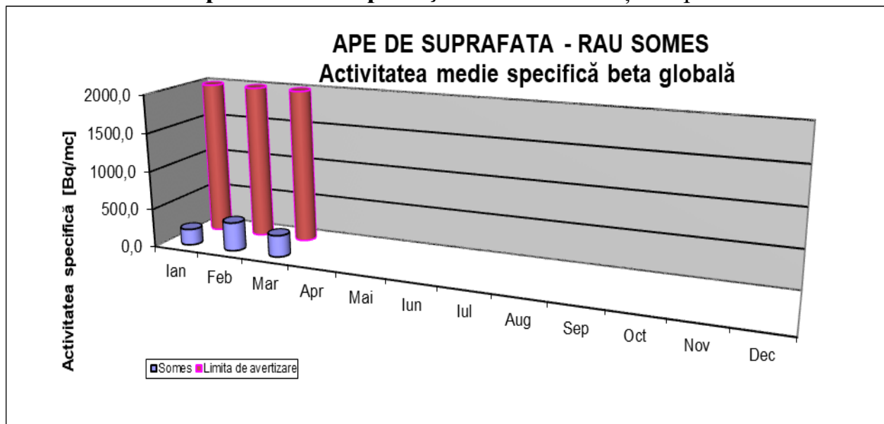
Fig. 2.3.6. Activitatea beta globală măsurată retard la 5 zile pentru apa de suprafață - Râul Someș
