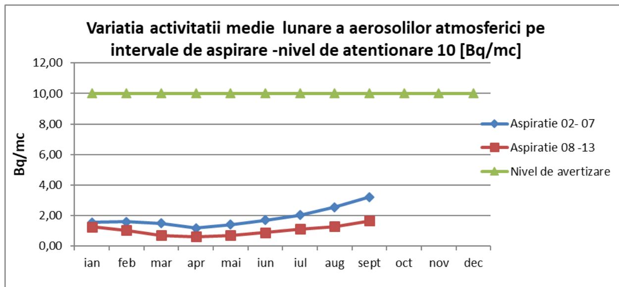
Fig. 2.3.1. Activitatea beta globală pentru aerosoli atmosferici
