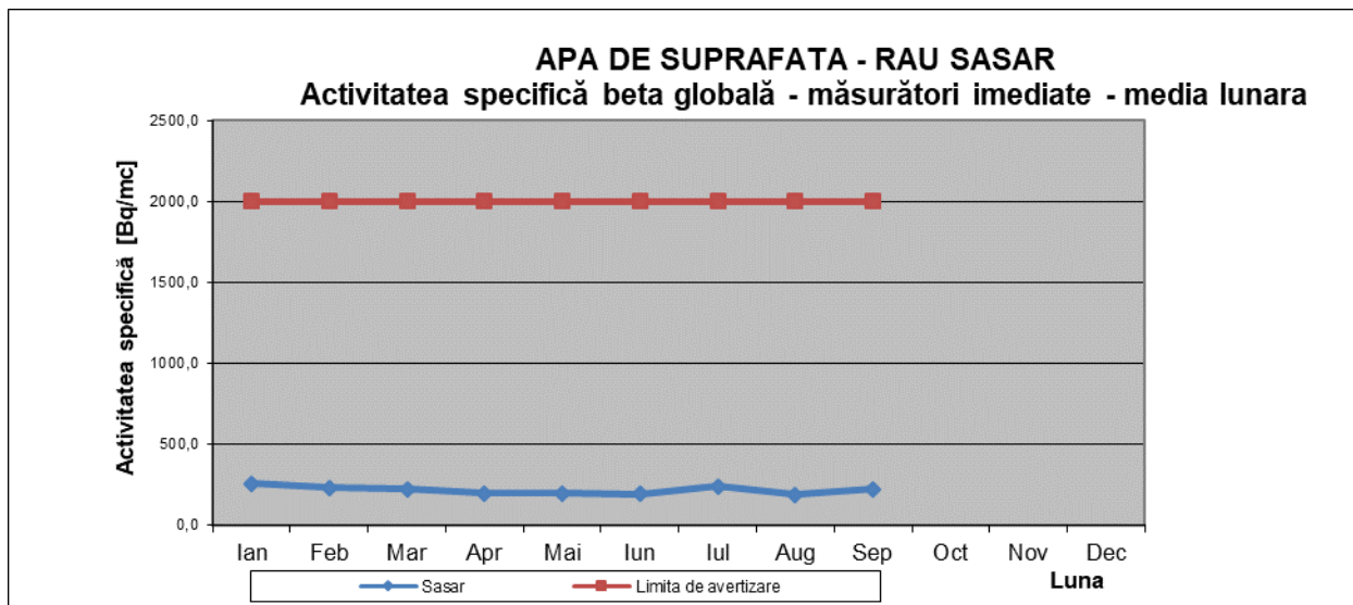
Fig. 2.4.5. Activitatea beta globală imediată pentru apa de suprafață din Râul Săsar (Pod Catedrală).
