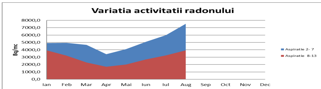
Fig. 2.3.2. Activitatea calculată a Radonului
