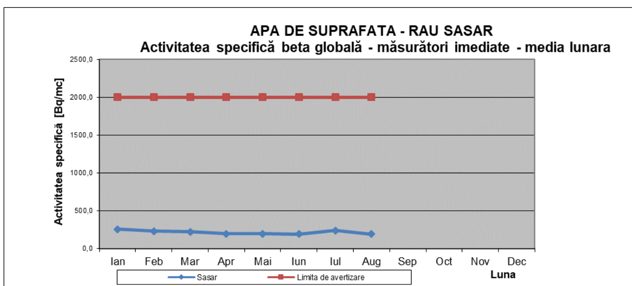
Fig. 2.4.5. Activitatea beta globală imediată pentru apa de suprafață din Râul Săsar (Pod Catedrala)
